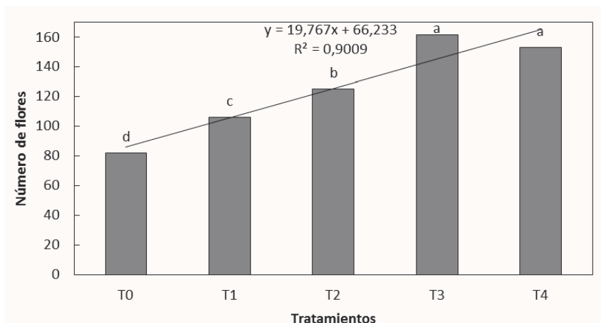
Figura 7.4. Producción de flores totales del cultivo de tomate en función a la cantidad de cal aplicada al suelo. Letras iguales no difieren estadísticamente según la prueba de tukey ( p=0,05 )
