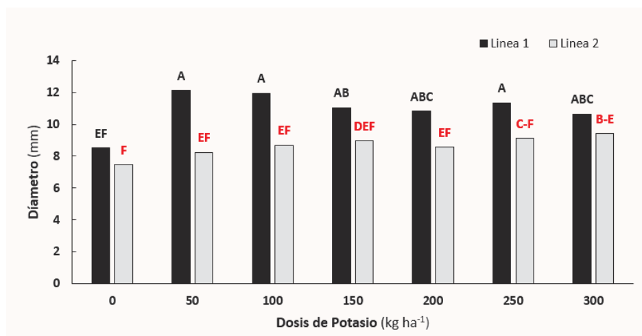
Figura 3. Comportamiento del diámetro de tallo de las dos líneas de batata ( Ipomoea batatas (L) Lam.) en relación con la dosis de Potasio aplicada bajo las condiciones climáticas del municipio de Sincelejo (Fuente: Elaboración propia).
