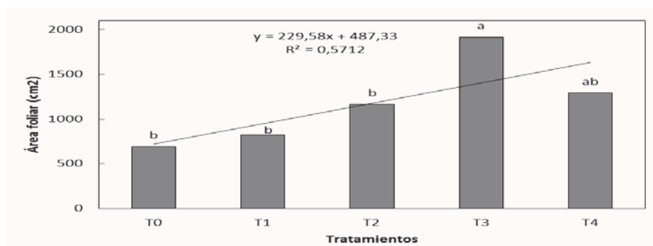
Figura 7.2. Área foliar. Letras iguales no difieren estadísticamente según la prueba de tukey ( p=0,05 )
