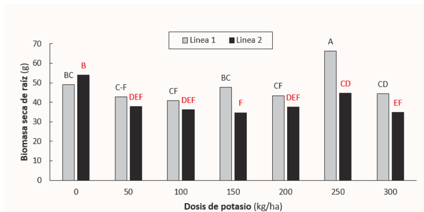
Figura 5. Comportamiento de la biomasa seca de raíces de las dos líneas de batata ( Ipomoea batatas (L) Lam.) en relación con la dosis de Potasio aplicada bajo las condiciones climáticas del municipio de Sincelejo (Fuente: Elaboración propia).
