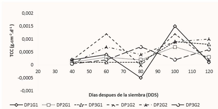
Figura 1.3. Tasa de crecimiento del cultivo (TCC) de dos genotipos de Batatas. (G1= Tainung y G2= Exportación), bajo tres distancias de siembra (DP1: 20 cm entre plantas, DP2: 50 cm entre plantas y DP3: 80 cm entre plantas) en el departamento de Sucre, Municipio de Morroa (2017).
