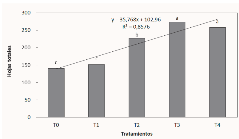
Figura 7.1. Hojas totales. Letras iguales no difieren estadísticamente según la prueba de tukey ( p=0,05 )
