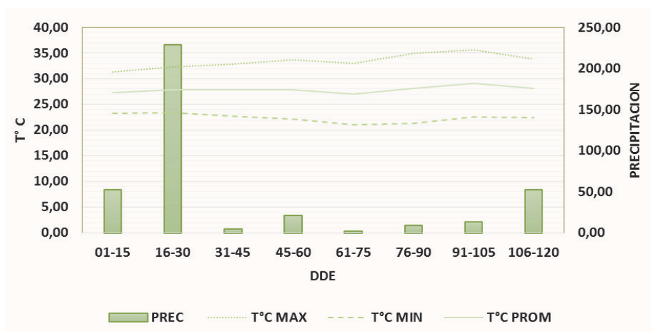
Figura 5.1. Condiciones ambientales presentes en el sitio de estudio durante el ciclo del cultivo de batata.
