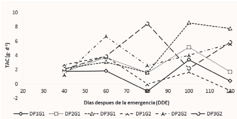
Figura 1.5. Tasa absoluta de crecimiento (TAC) de dos genotipos de Batatas (G1= Tainung y G2= Exportación), bajo tres distancias de siembra (DP1: 20 cm entre plantas, DP2: 50 cm entre plantas y DP3: 80 cm entre plantas) en el departamento de Sucre, Municipio de Morroa (2017).
