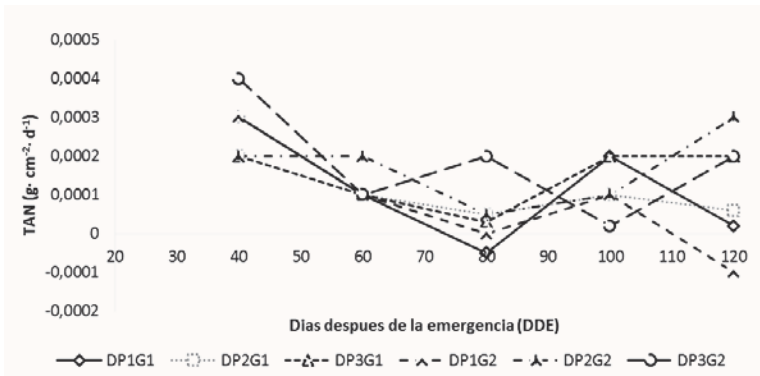
Figura 1.2. Tasa de asimilación neta (TAN) de dos genotipos de Batatas. (G1= Tainung y G2= Exportación), bajo tres distancias de siembra (DP1: 20 cm entre plantas, DP2: 50 cm entre plantas y DP3: 80 cm entre plantas) en el departamento de Sucre, Municipio de Morroa (2017)
