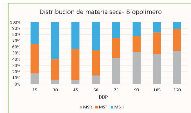
Figura 4.2. Distribución porcentual de materia seca en hojas (MSH), tallo (MST) y raíces tuberosas (MSR) del cultivo de batata medida cada 15 días después del prendimiento (DDP) hasta 120 DDP, aplicándole diferentes tipos de fertilizantes y un tratamiento testigo.
