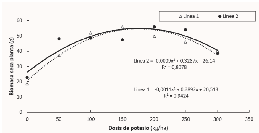
Figura 4. Tendencia en la variable biomasa seca aérea de las dos líneas de batata ( Ipomoea batatas (L) Lam.) en relación con la dosis de Potasio aplicada bajo las condiciones climáticas del municipio de Sincelejo (Fuente: Elaboración propia).
