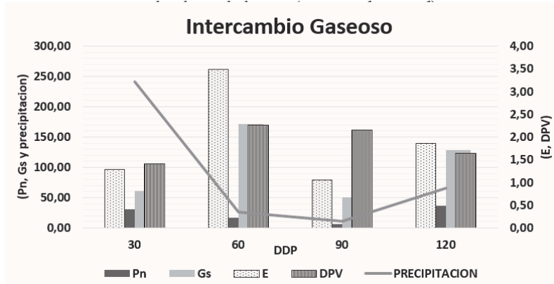
Figura 4.1. Intercambio gaseoso mensual vs. condiciones ambientales (precipitación) en el cultivo de batata.
