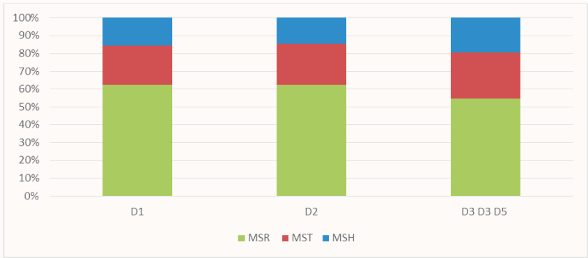
Figura 6.2. Distribución de materia seca por órganos de las plantas de batata, materia seca de raíces (MSTR: %), tallos (MST: %) y hojas (MSH: %). D1: sin aplicación edáfica HC (0,00 g planta -1 ); D2: aplicación edáfica de 25 kg ha -1 de HC (1 g planta -1 ); D3: aplicación al suelo de 90 kg ha -1 de H (3,6 g planta -1 ); D4: aplicación al suelo de 155 kg ha -1 de HC (6,2 g planta -1 ); D5: aplicación al suelo de 220 kg ha -1 de HC (8,8 g planta -1 ). CONTR = contraste. ns: no significativo *: Significativo al 5%; ** significativo al 1%.
