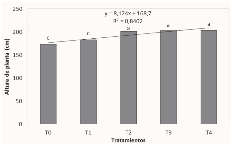
Figura 7.3. Efecto de la aplicación de cal en la altura de la planta de tomate. Letras iguales no difieren estadísticamente según la prueba de tukey ( p=0,05 )
